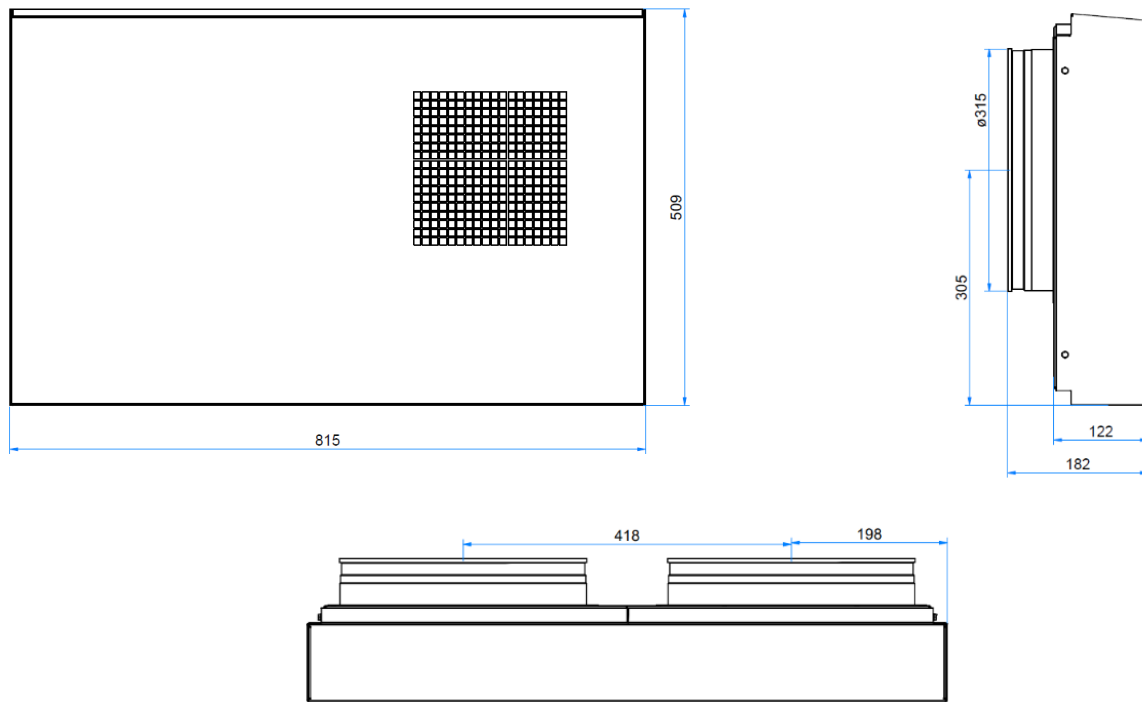
Bild 2: Måltritning för vägghuv
